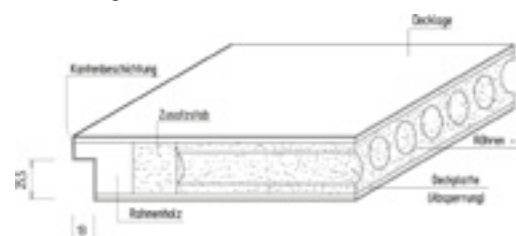
Innenleben einer Röhrenspantür
