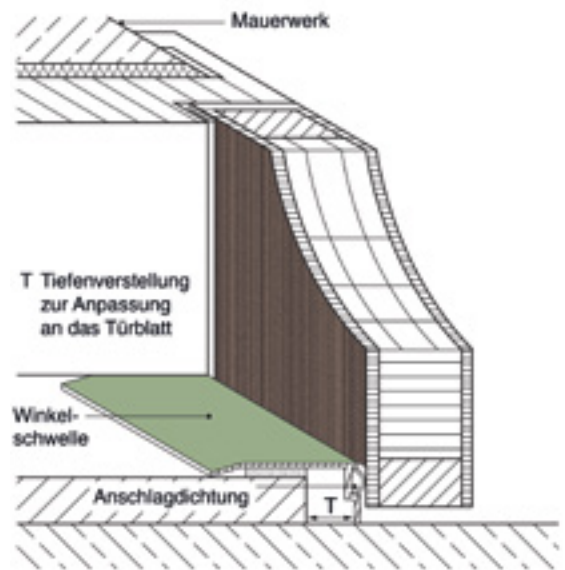
Anschlagsschwelle
