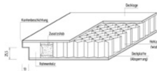
Innenleben einer Wabentür
