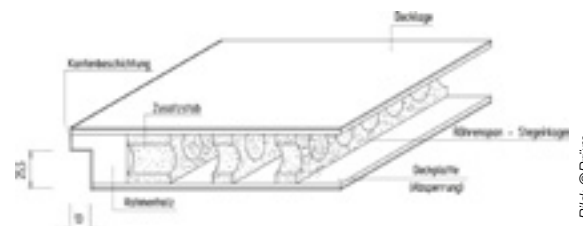
Innenleben einer Röhrenspanstreiftür
