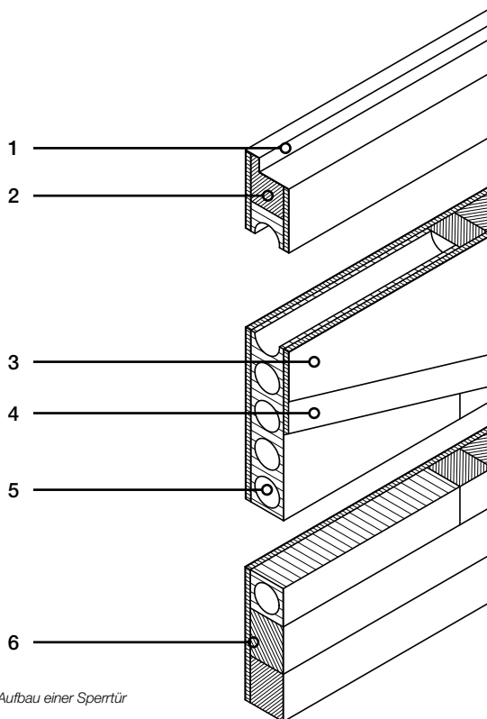
Innenleben einer Röhrenspanstreiftür
