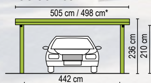
Modell „Burg M (T), Select“, Abb. zeigt Sonderausstattung
