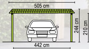
Modell „Glücksburg M (T)“, Natur – Abbildung zeigt Sonderausstattung
