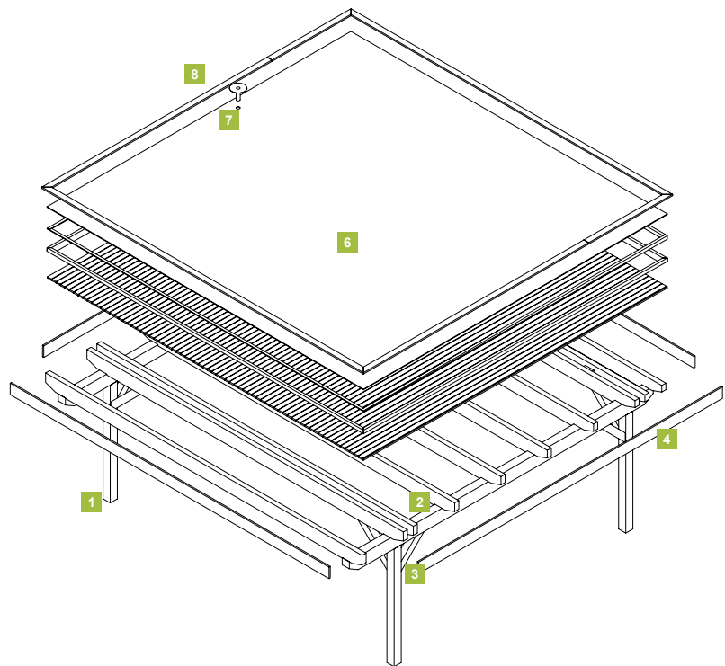
Explosions-Detail: Flachdach mit Foliendach und integriertem Foliendach-Ablauf
