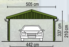
Modell „Walsrode M (D), Select“, Gestaltungsbeispiel mit Geräteraum Typ 03 und Querkopfbänder – Gestaltungsbeispiel
