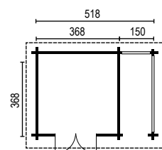
368×368 cm + 150 cm mit seitlich integriertem Unterstand, mit 45 mm BB
