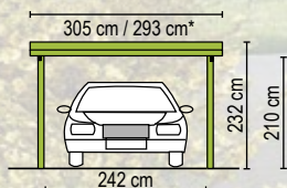
Modell „Bergen K (T), Classic“, Abb. zeigt Gestaltungsbeispiel mit Sonderausstattung Pfostenbögen
