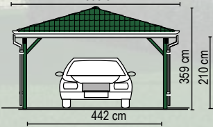
Modell „Kiel M (D), Master“ mit Geräteraum Typ 09 und bauseitiger Zinkrinne
